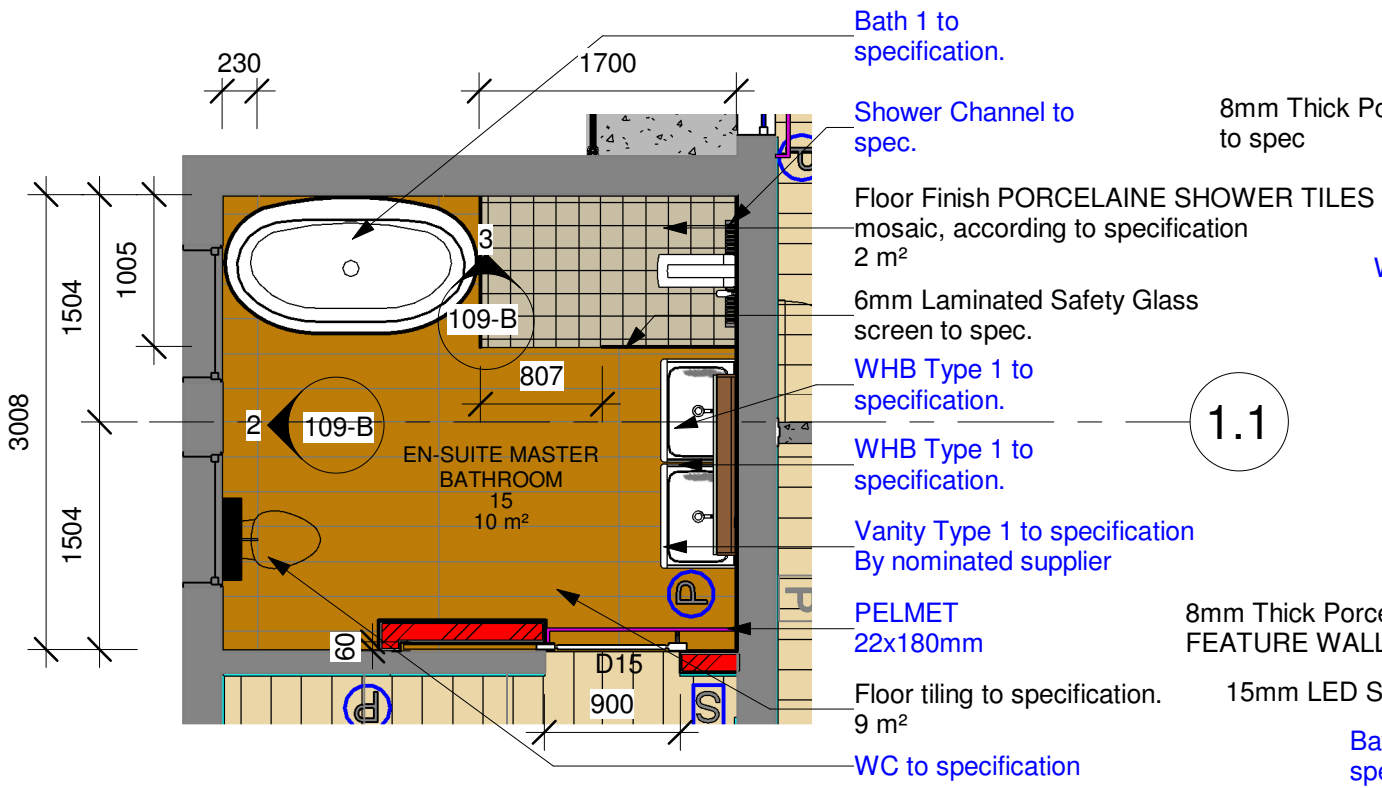
1 FIRST FLOOR - Main En Suite 1 : 50
